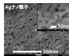
図2 二次電子像(サンプル：樹脂基板上のAgナノ粒子 Ptコーティング有)
